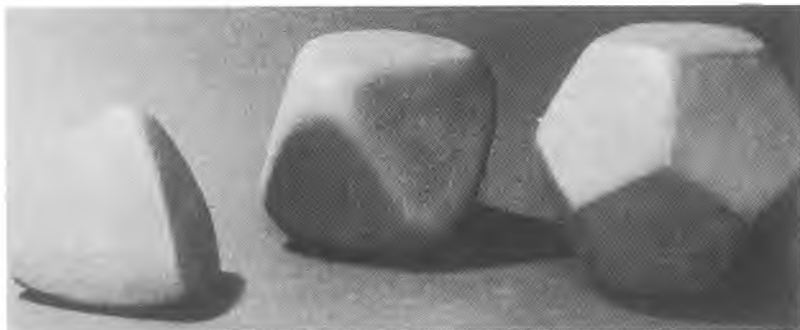
● Från vänster tetraeder, oktaeder och pentagondodekaeder
